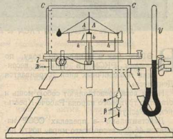
Рис. 6. Микро-весы Стиля и Гранта.
