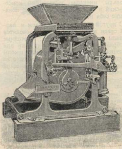
Рис. 4. Элеваторные весы для зерна.
